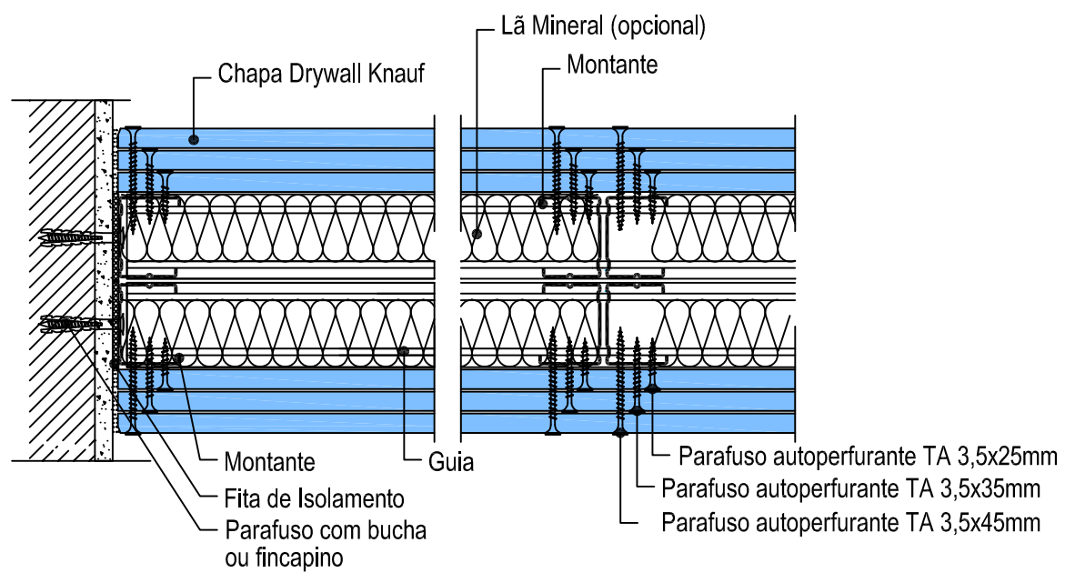
DETALHE - PAREDE W116 COM MONTANTE DUPLO
