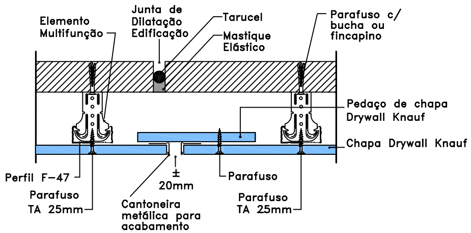
1 CORTE HORIZONTAL – JUNTA DE DILATAÇÃO EM W623 SEM ESCALA
