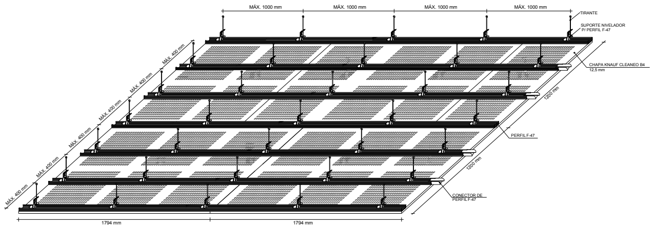
PERSPECTIVA CLEANEO B4 ESC: 1/10
