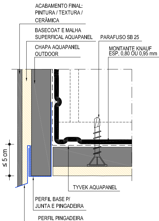
3 DETALHE B - Corte S/ ESCALA
