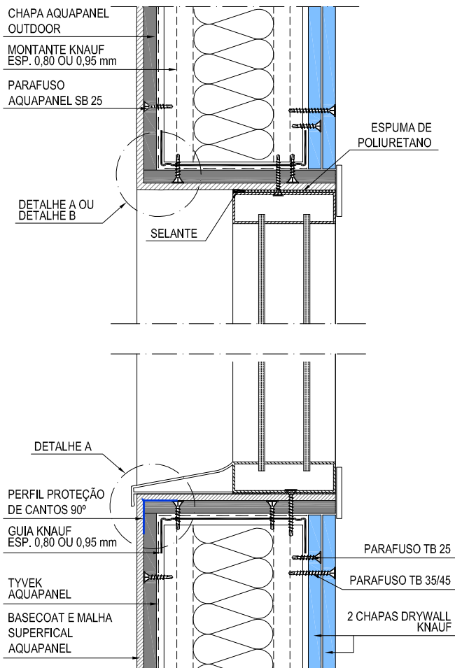
1 PAREDE - JANELA - Corte ESCALA 1:5
