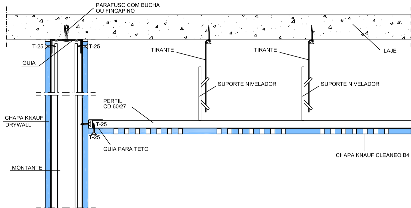
CORTE LONGITUDINAL CLEANEO B4
