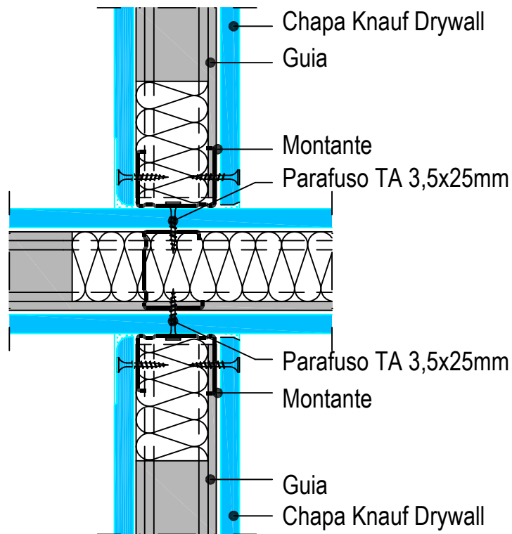
1 CORTE HORIZONTAL COM ENCONTRO EM CRUZ- W111 SEM ESCALA
