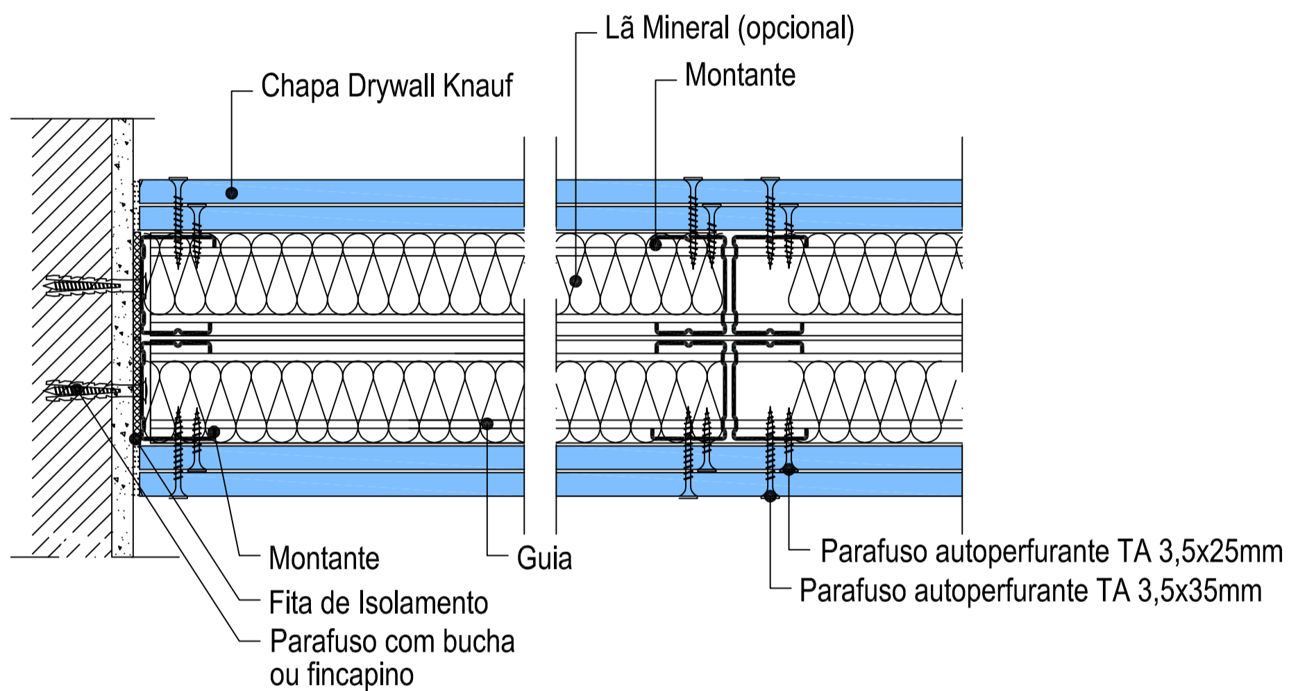
DETALHE - PAREDE W116 COM MONTANTE DUPLO
