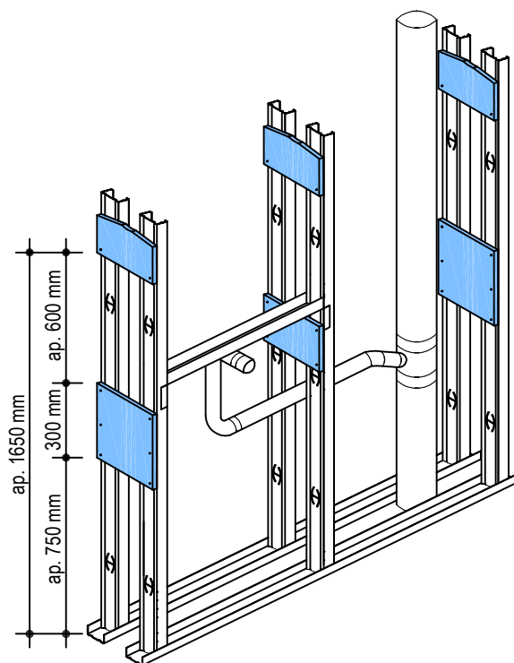
DETALHE - INSTALAÇÕES HIDRÁULICAS
