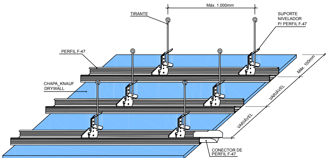
1 PERSPECTIVA - TETO D112 UNIDIRECIONAL COM PERFIL F-47 E 1 CHAPA SEM ESCALA
