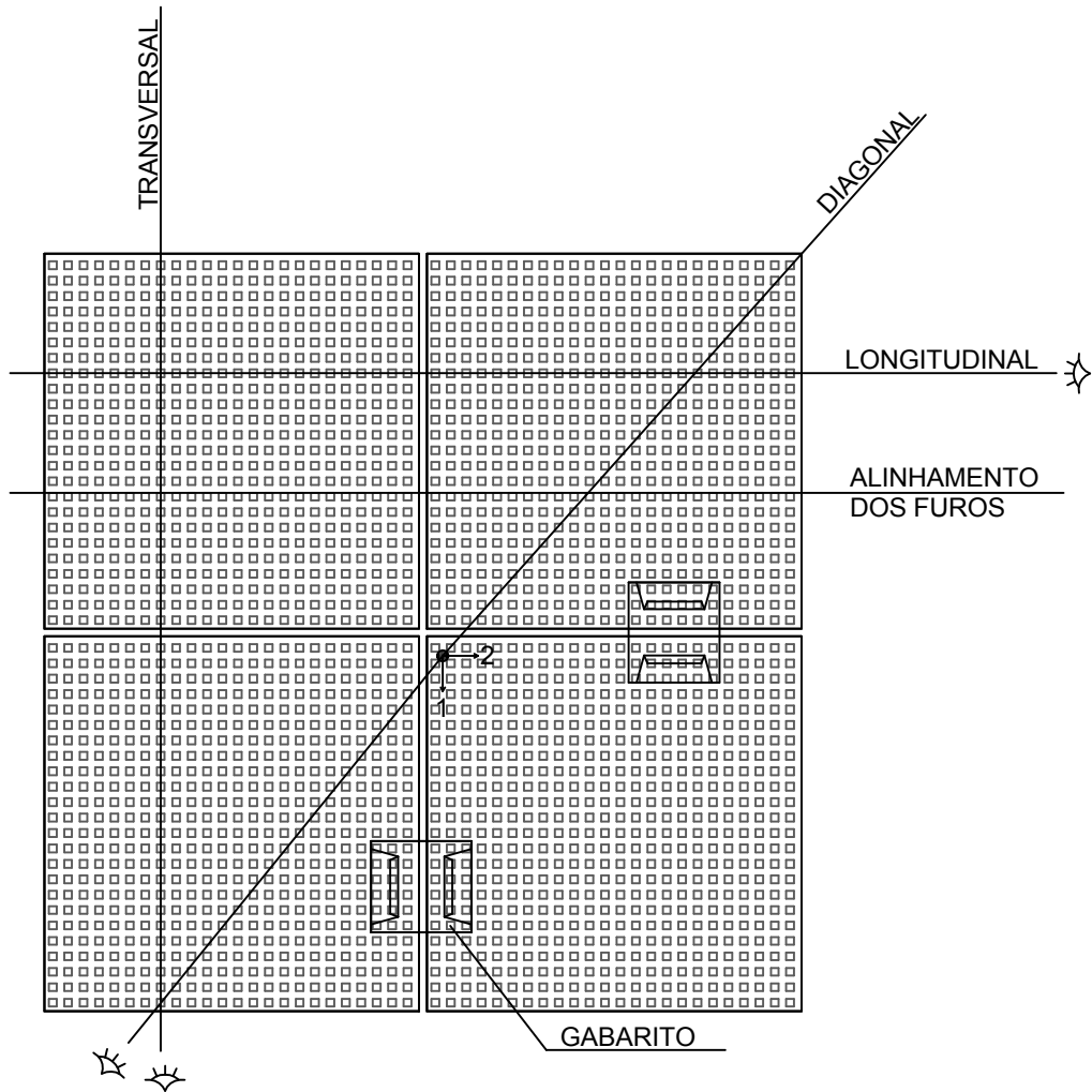
ESQUEMA DE MONTAGEM - CLEANEO sem escala
