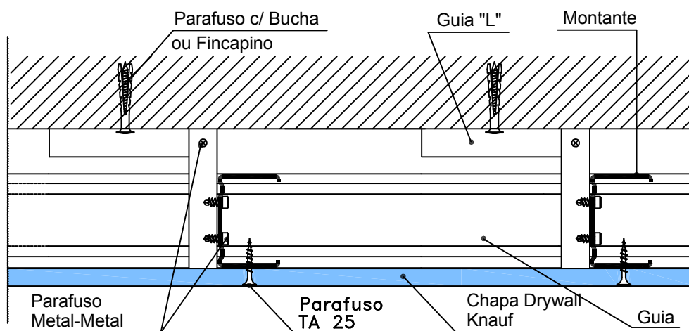
1 DETALHE - CORTE HORIZONTAL - REVESTIMENTO W623 SEM ESC.
