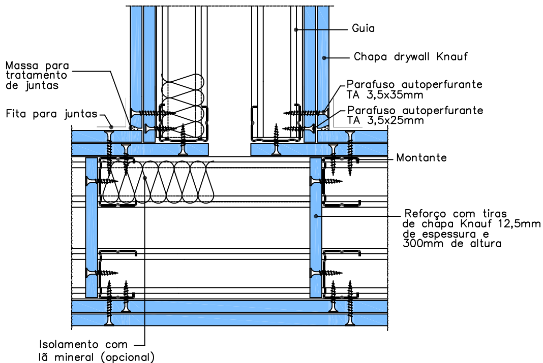
1 DETALHE – ENCONTRO DE PAREDE EM T – W116 SEM ESCALA
